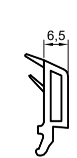
Штапик под с/п. 42мм арт. 6004
