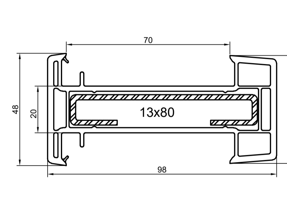
Статический усилитель арт. 8188 ( 118 )
