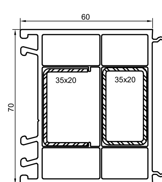
Расширитель 70x60мм арт. 8176 ( 629600 )
