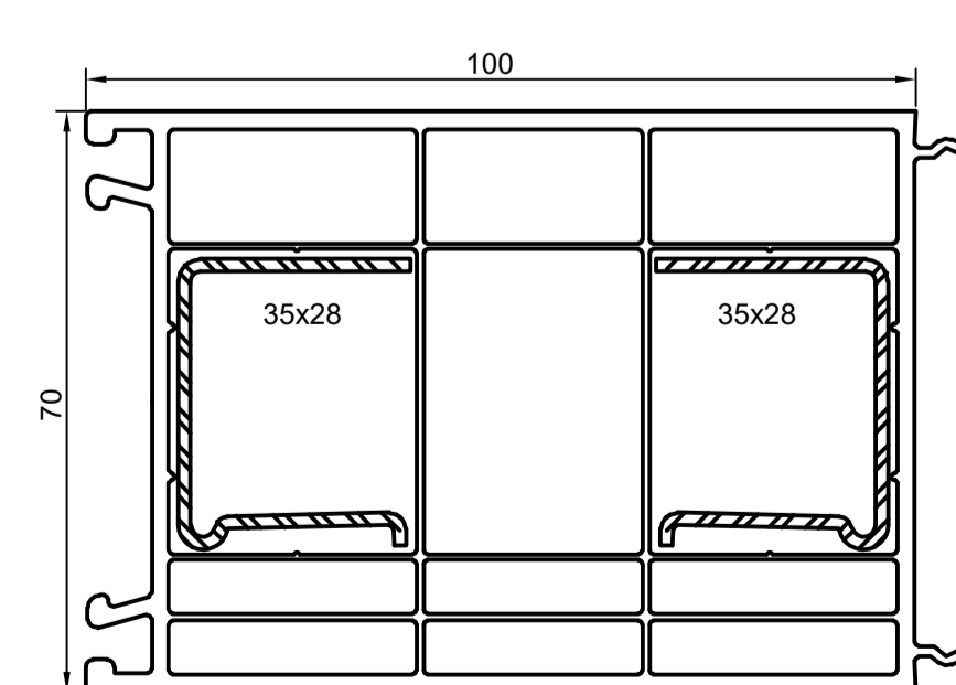
Расширитель 70x100мм арт. 8170 ( 629100 )
