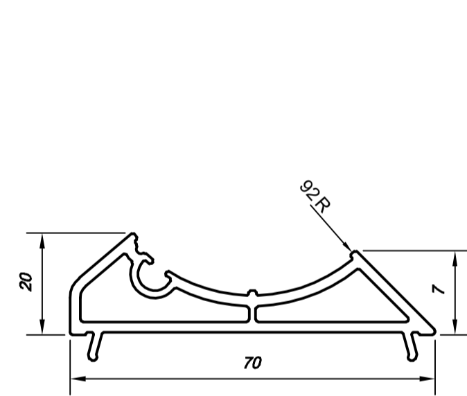
Адаптер эркера арт. 8181 ( 110 )
