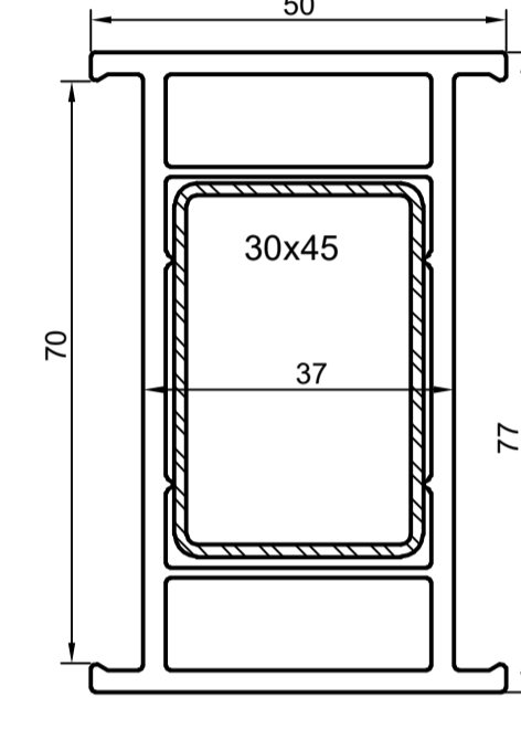
Соединитель (расширитель 70x37) арт. 8171 (111)
