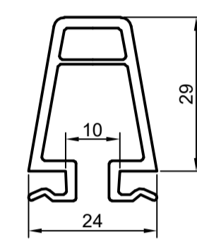
Профиль соединителя арт.8082
