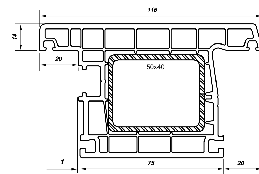
Створка дверная наружного открывания Т арт. 8150
