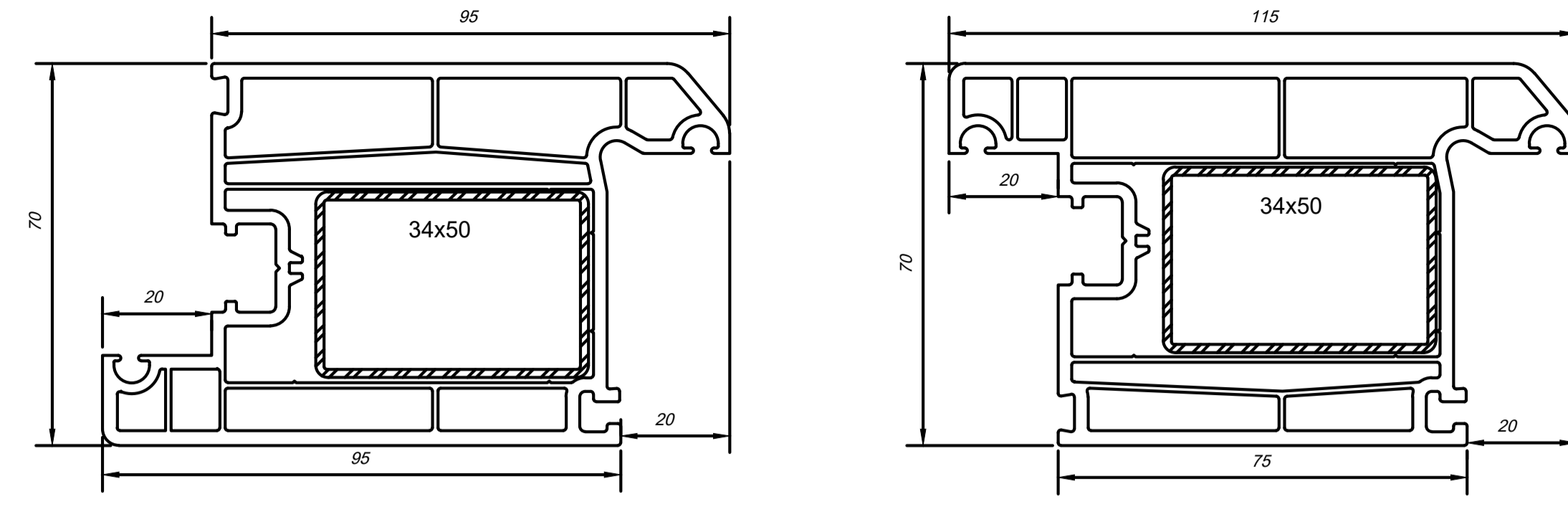
Створка внутреннего открывания Z арт. 104
