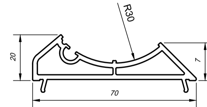
Адаптер эркера арт. 110
