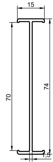
Соединитель 70 арт. 109
