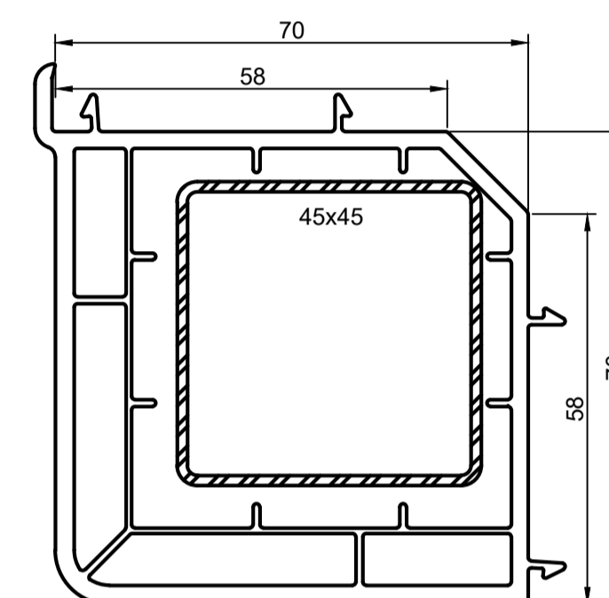
Соединитель угловой 90° арт. 112
