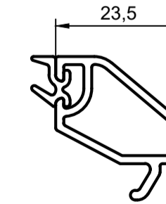
Штапик под с.п. 24мм арт. 108
