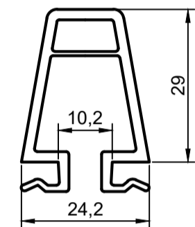
Профиль соединителя арт. 8082
