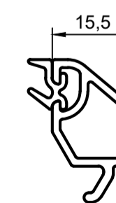
Штапик под с.п. 32мм арт. 107
