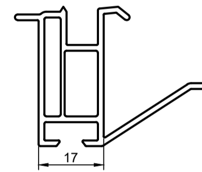
Подставочный арт. 201
