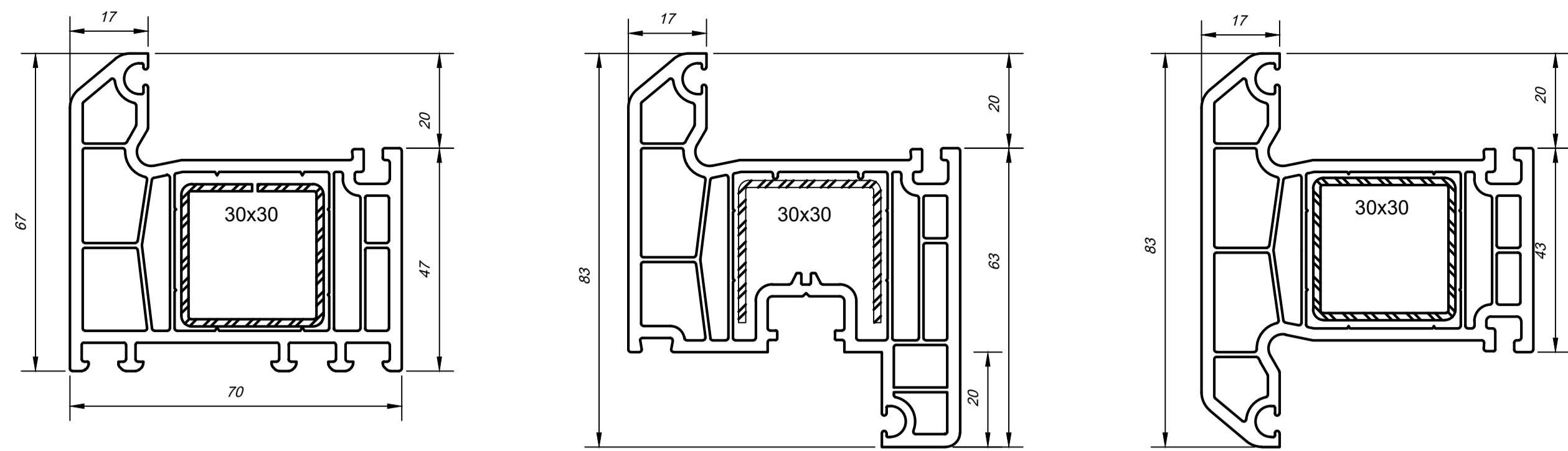
Рама арт. 101
