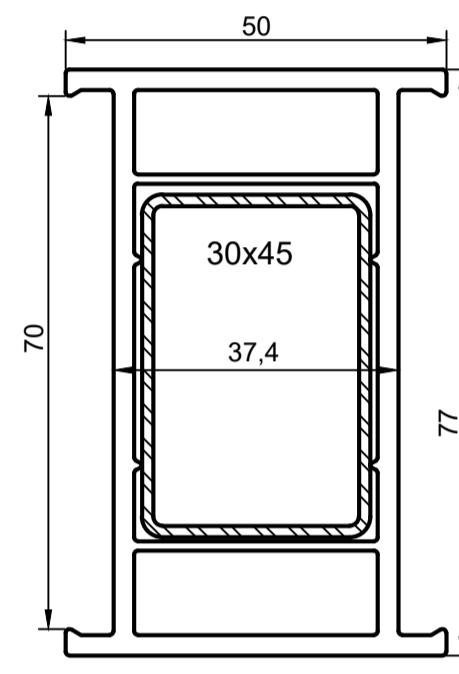
Соединитель (расширитель 70x37) арт. 111
