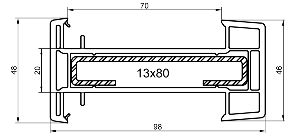
Статический усилитель арт. 118
